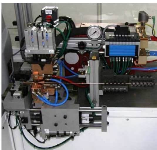
Tête de compactage et système d'avance
