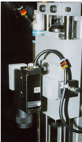
CAPTEUR MONTE SUR COULISSEAU POUR CONTROLE PRESENCE DEPOT DE BRASURE
