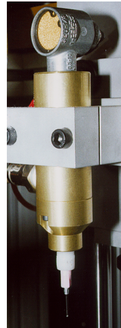
VALVE DE DISTRIBUTION DE BRASURE MONTEE SUR COULISSEAU
