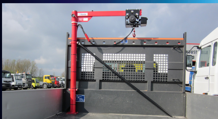
Montage benne.
