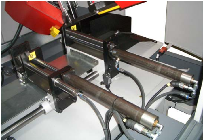
Étau principal et étau avance-barre
