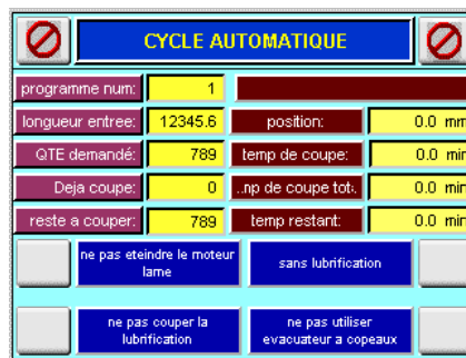
Exemple du menu sur l'écran tactile couleur
